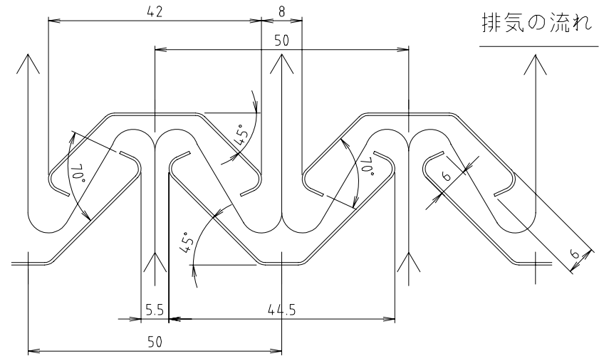
衝突板断面
