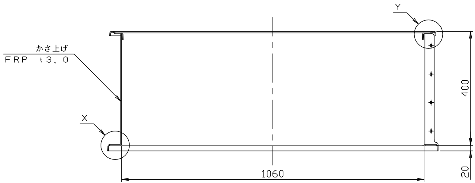
AA' 断面
