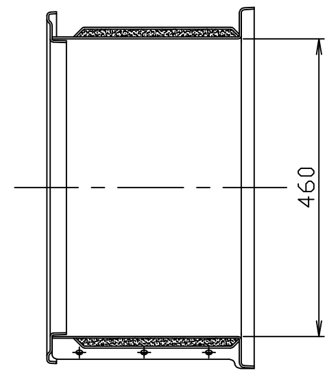
BB' 断面
