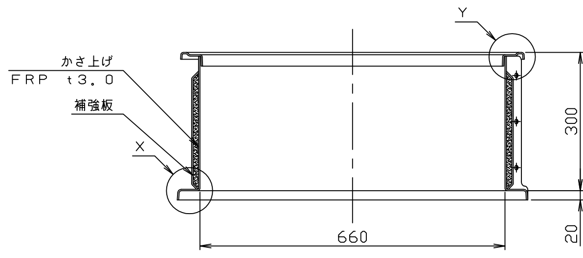
AA' 断面
