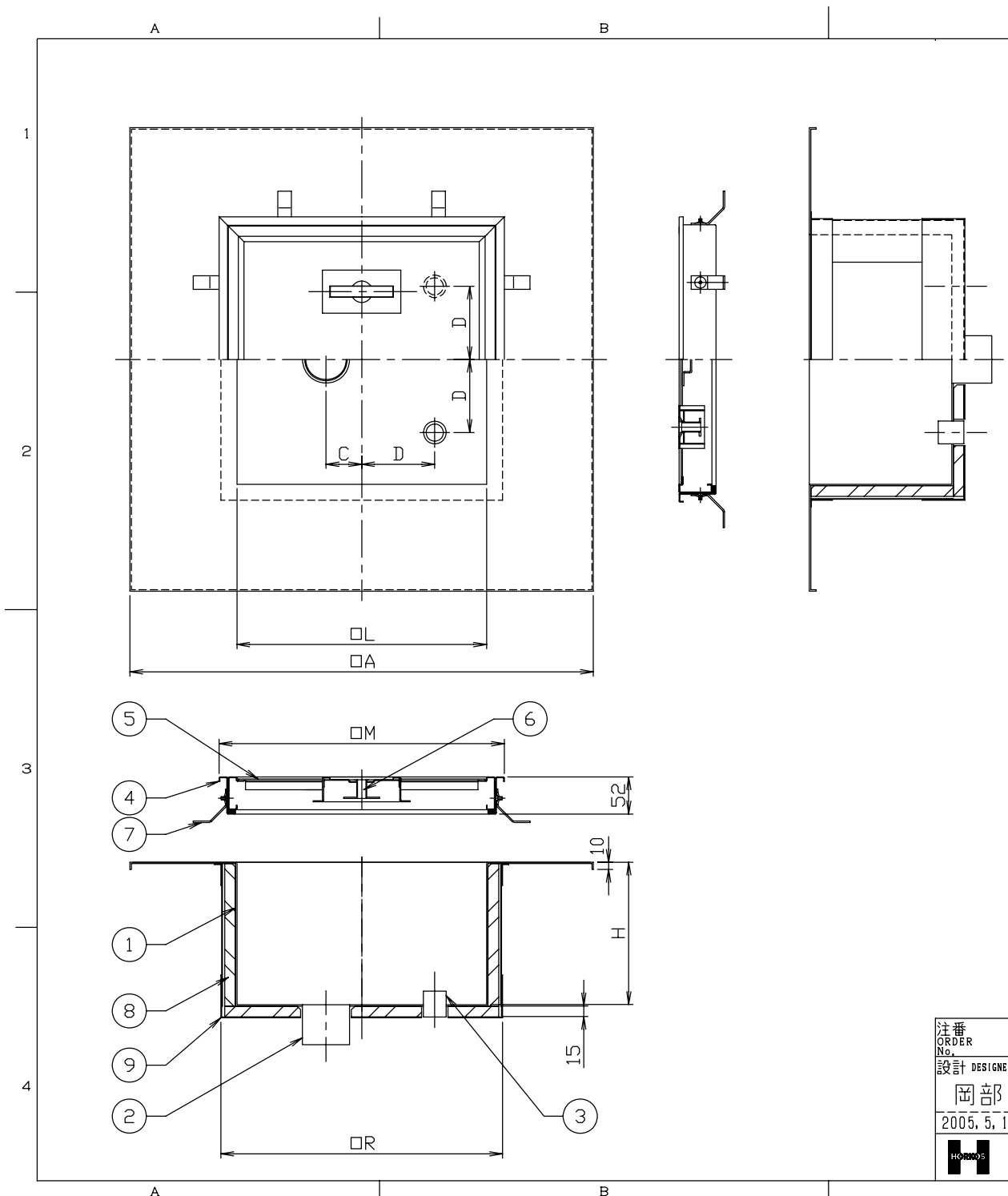
寸法表
