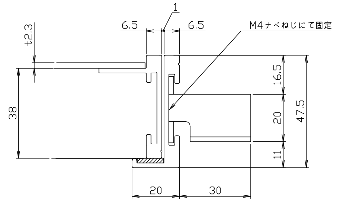
枠断面詳細
