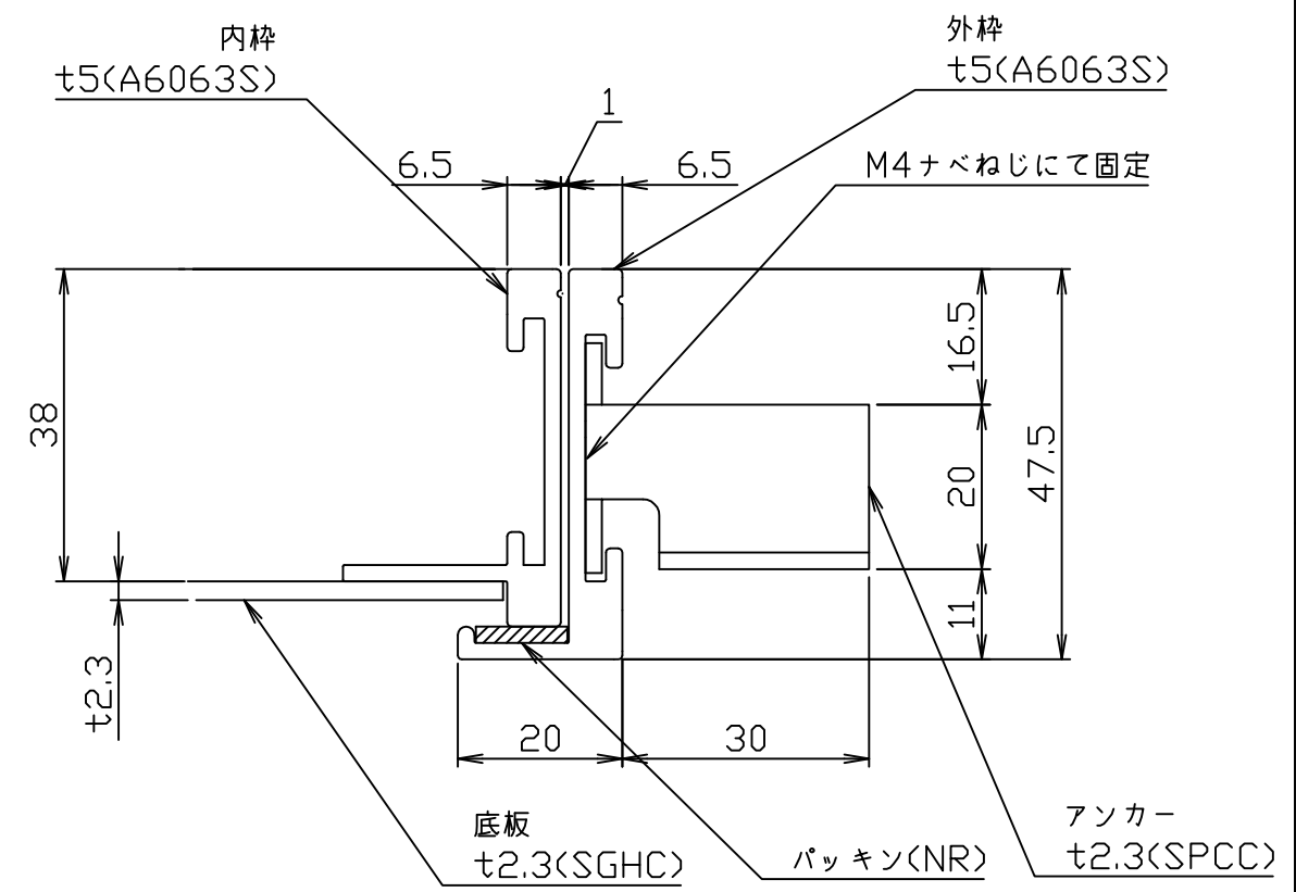
枠断面詳細
