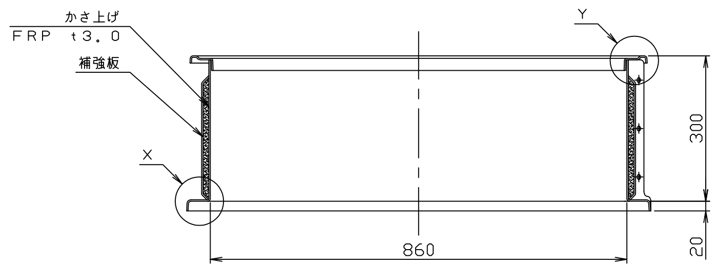
AA' 断面
