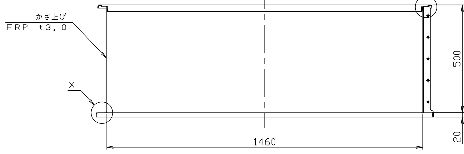
AA' 断面
