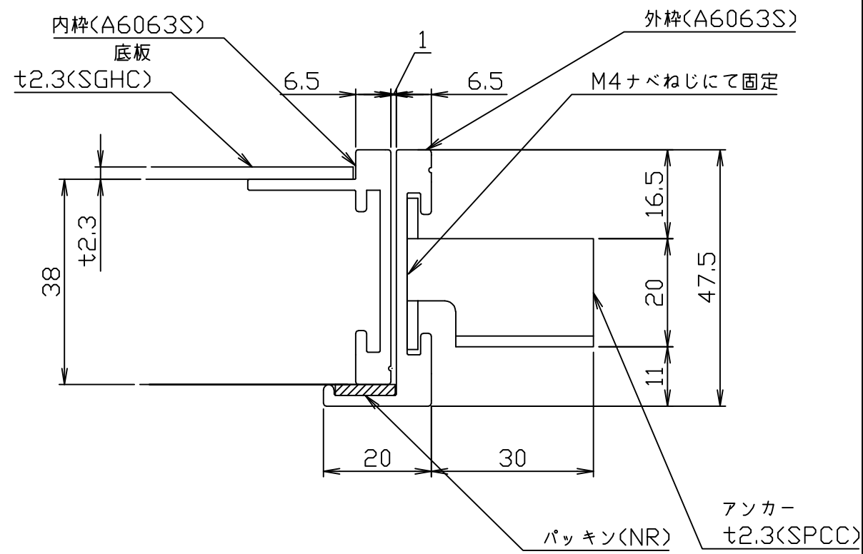
枠断面詳細
