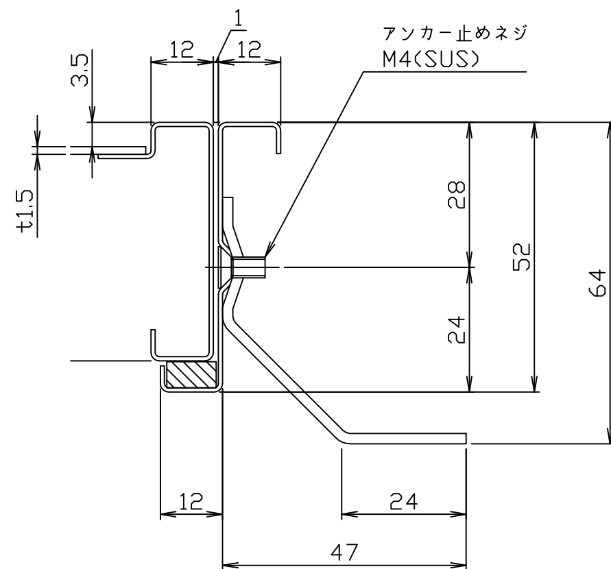
断面詳細
